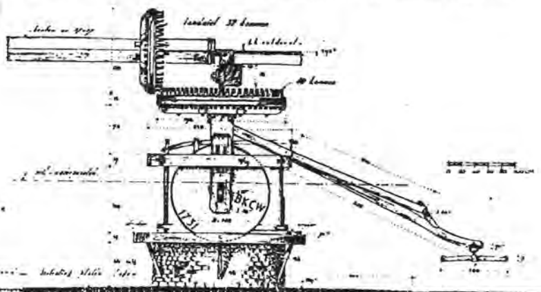
Schets van een rosmolen, vooraanzicht. (Deze tekening en de foto op blz. 8 zijn uit het boek van A.J. Bernet Kempers: "Oliemolens", uitgegeven door het Rijksmuseum voor Volkskunde, Arnhem en uitg. Terra te Zutphen.
