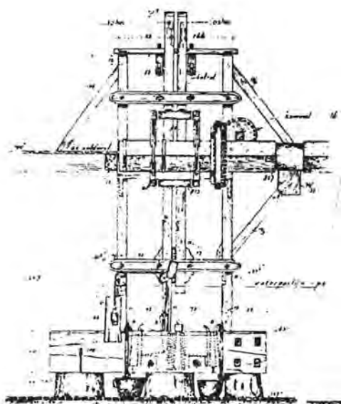
Schets van een rosmolen, vooraanzicht. (Deze tekening en de foto op blz. 8 zijn uit het boek van A.J. Bernet Kempers: "Oliemolens", uitgegeven door het Rijksmuseum voor Volkskunde, Arnhem en uitg. Terra te Zutphen.
